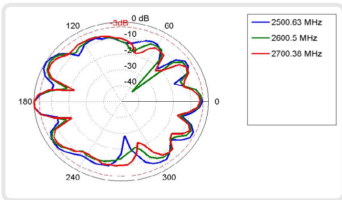
H-Plane: 2500 - 2700 MHz
