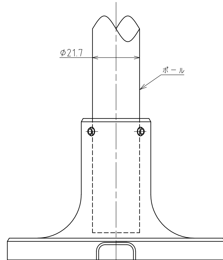
取付参考図 (Reference Drawing)
